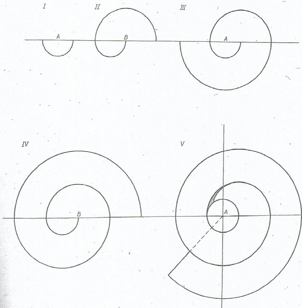
Rys. 107. Wolant z żabotem krojony w kształcie spirali – rysunek żurnalowy i konstrukcyjny w etapach I÷V
