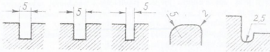
Rys. 60. Sposoby wpisywania małych wymiarów
