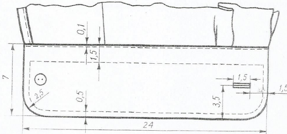
Rys. 61. Wymiarowanie rysunku technicznego mankietu do koszuli
