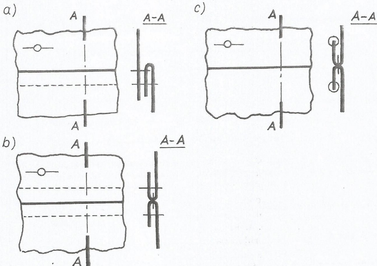
Rys. 67. Szew zwykły: a) przelozony, przestebnowany, b) rozlozony, rozstebnowany, c) rozlozony, brzegi obrzucone
