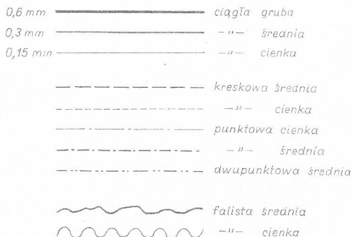
Rys. 21. Linie rysunkowe
